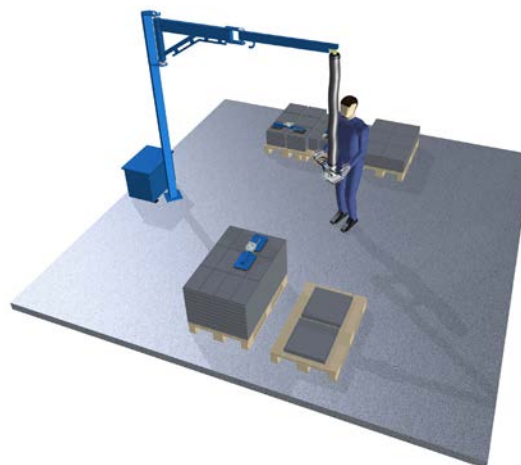
Viksvingkranar, fasta och mobila.
